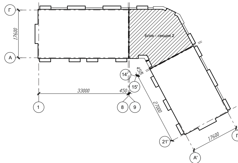
Компоновочная схема
