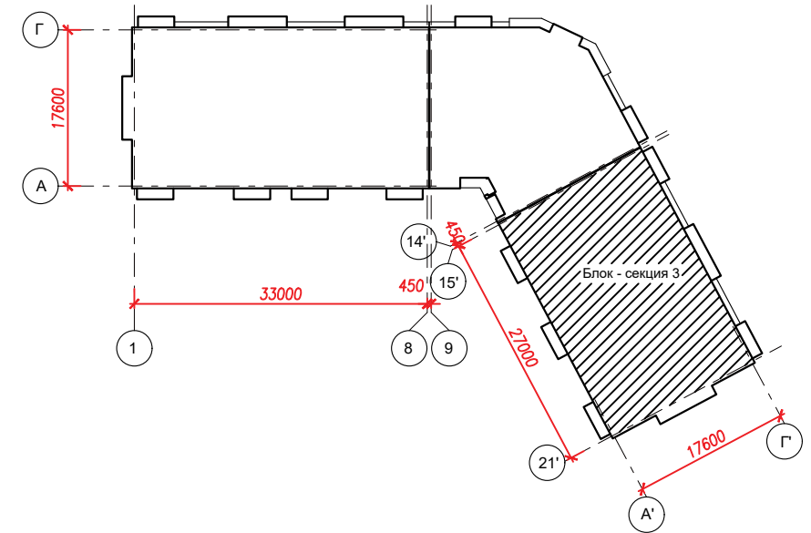
Компоновочная схема
